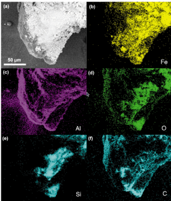
図15:メチルエチルケトンで処理した後の赤い層の走査電子顕微鏡写真と、XEDSによる鉄、アルミニウム、酸素、珪素、炭素の元素マップ
