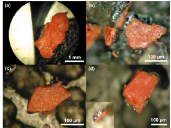
未着火のアルミノ・テルミット剤:2層の薄板片
