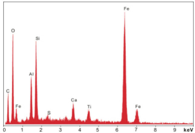
図25:「DSCの中で赤と灰色の薄板片を発火させて作られる球体、およびその典型的なXEDSスペクトル」
