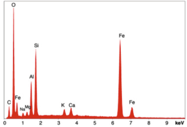
図24:「市販のテルミットの発火で作られる球体、およびその典型的なXEDSスペクトル」
