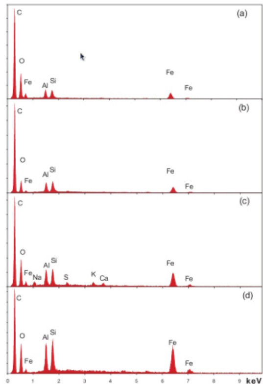
(右) 図6:4つのWTCの塵埃サンプルにある赤い層から得られるXEDSによる元素のスペクトル
