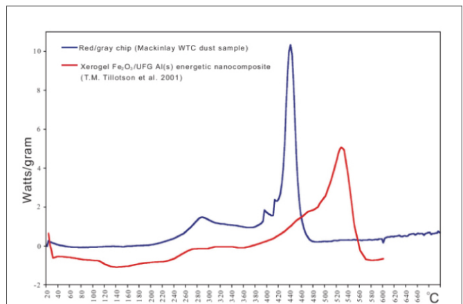
図29:青い線はサンプル1のDSCトレースで、Xerogel Fe 2 O 3 /UFG Al nanocomposite (Tillotson他)と比較されている。どちらのDSCトレースでも、反応が560°C未満で起こっていることが分かる。
