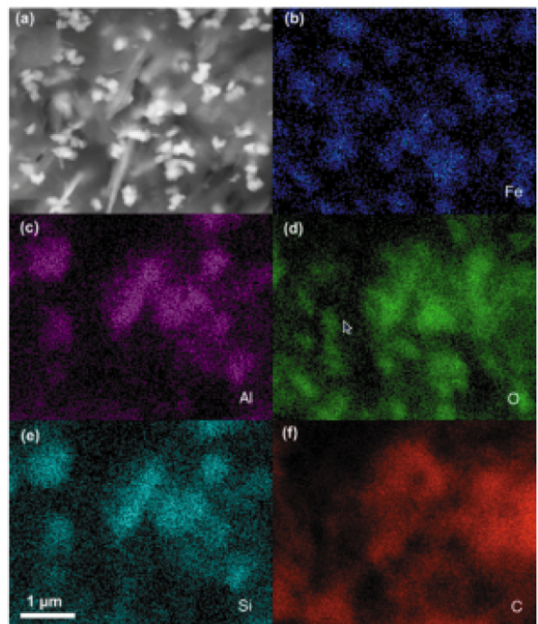
図10:処置以前の赤い層の走査電子顕微鏡写真と、XEDSによる鉄、アルミニウム、酸素、珪素、炭素の元素マップ
