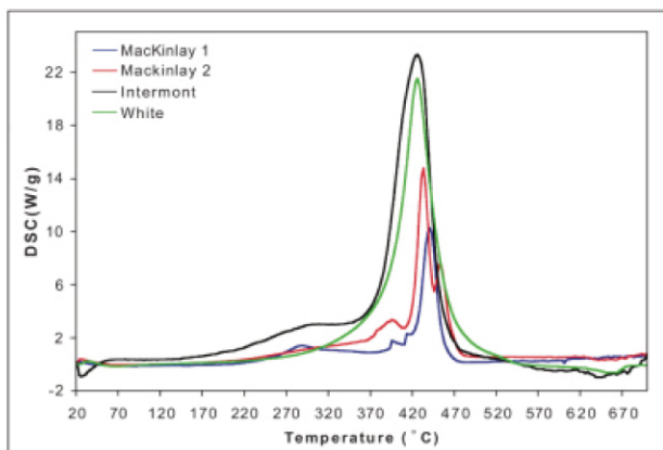
図19:4つのサンプルのそれぞれから採られた薄板片のDSCトレース
