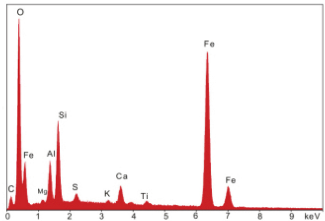
図27, 28:「WTCの塵から採られた小球」そして「WTCの塵で見つかった小球のXEDSスペクトル」
