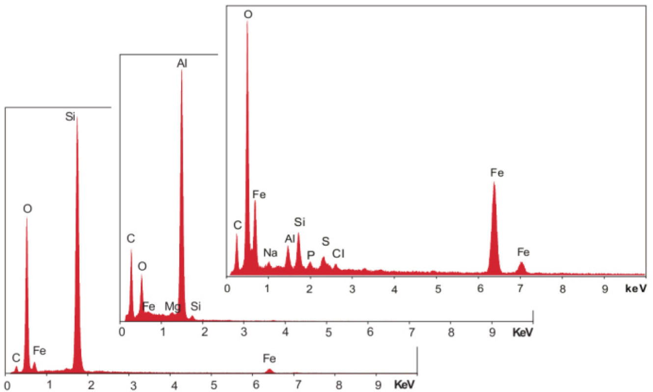
図16、図17、図18のコラージュ。後ろ側から手前側に向かって、それぞれのグラフに次のような説明がついている。「メチルエチルケトンで処理した赤い物体にある赤い他孔質の基盤で珪素に富む箇所から得られるXEDSスペクトル」、「メチルエチルケトンに漬けられた赤い薄板片のアルミニウムに富む箇所から10kVで検出できるXEDSスペクトル」、「メチルエチルケトンに漬けられた赤い薄板片の鉄を多く含む部分から15kVの電子ビームによって検出されるXEDSスペクトル」。
