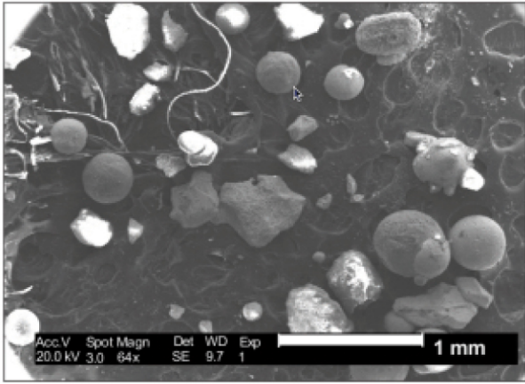
図24:「市販のテルミットの発火で作られる球体、およびその典型的なXEDSスペクトル」
